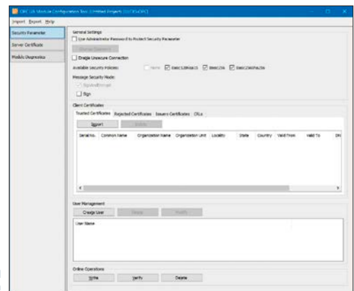
OPC UA Module Configuration Tool Security parameter settings screen
